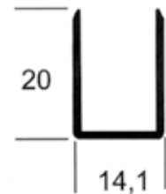
M - 24 0,175 kg/m
