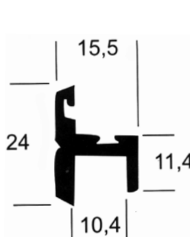
M - 8 0,304 kg/m
