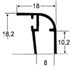
M - 72 0,158 kg/m
