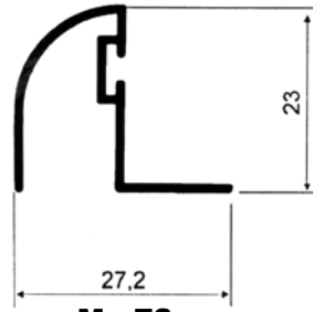
M - 73 0,240 kg/m
