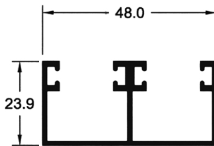
M - 6/B (10mm) 0,633 kg/m
