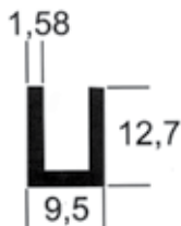
M - 20 0,129 kg/m
