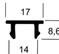
M - 9 0,119 kg/m
