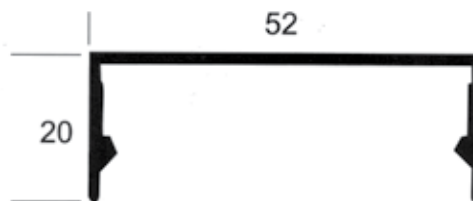
M - 64 0,351 kg/m
