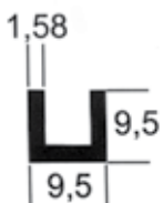
M - 21 0,108 kg/m
