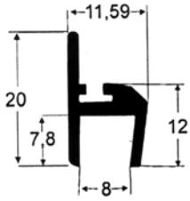
M - 71 0,168 kg/m
