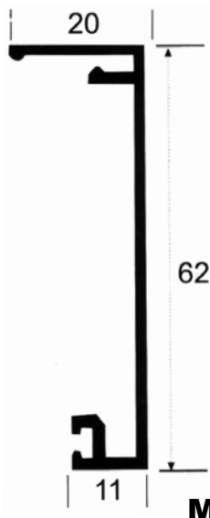
M - 5 0,550 kg/m
