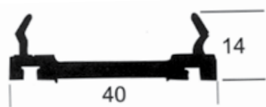
M - 29 0,380 kg/m
