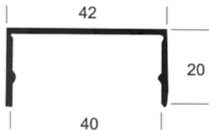
M - 28 0,265 kg/m
