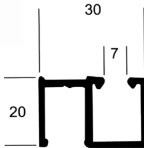
M - 14 0,304 kg/m
