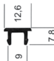
M - 57 0,099 kg/m
