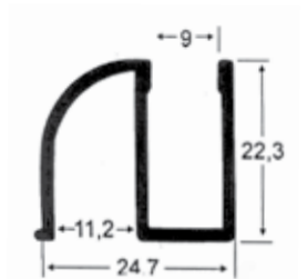
M - 69 0,289 kg/m
