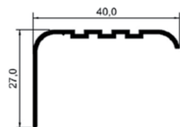
ME - 013 0,323 kg/m
