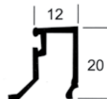
M - 41 0,195 kg/m
