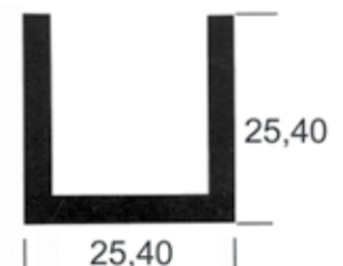
U - 1'' 0,490 kg/m
