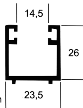
M - 6 0,371 kg/m
