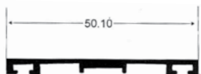
M - 75 0,380 kg/m
