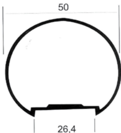
M - 63 1,811 kg/m
