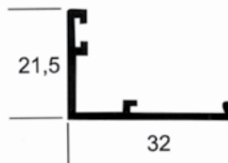
M - 40 0,270 kg/m
