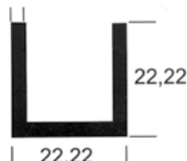
M - 16 0,400 kg/m
