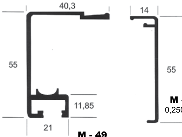
M - 49 0,790 kg/m
