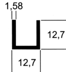
M - 19 0,151 kg/m
