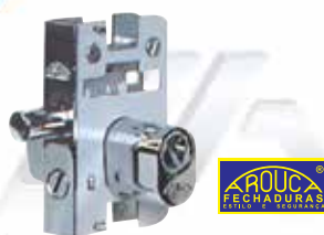
Miolo para fechadura
