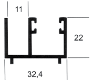
M - 55 0,500 kg/m
