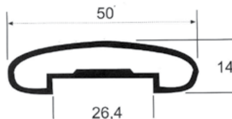
D - 095 0,544 kg/m
