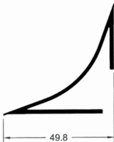
TSL - 003 0,833 kg/m
