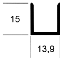
M - 60 0,132 kg/m
