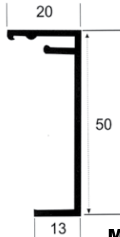
M - 4 0,344 kg/m
