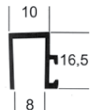
M - 11 0,200 kg/m
