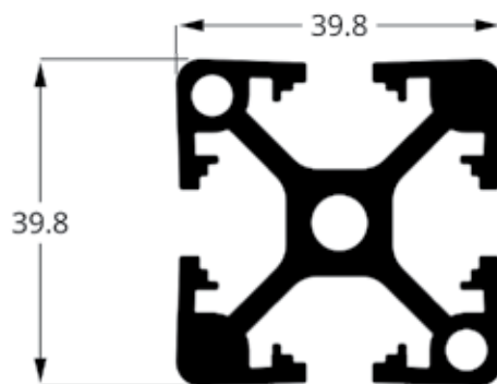
PERFIL ESTRUTURAL
