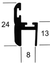
M - 56 0,309 kg/m
