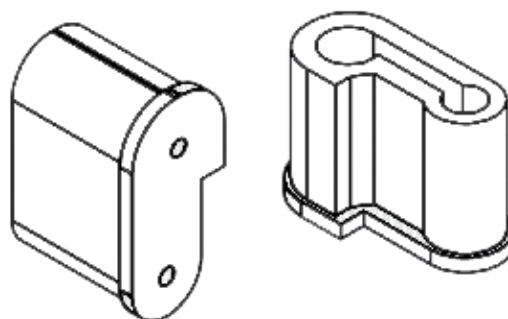
SAPATA FIXAÇÃO (DV 300)
