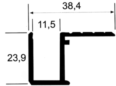
M - 7 0,436 kg/m
