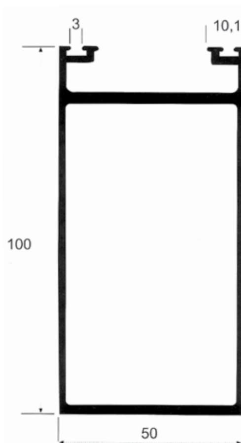
M - 66 1,989 kg/m
