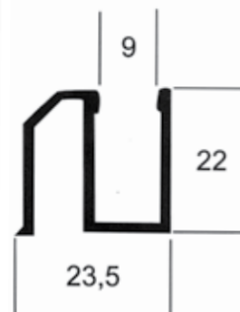
M - 58 0,302 kg/m
