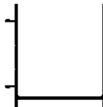
M - 84 0,592 kg/m
