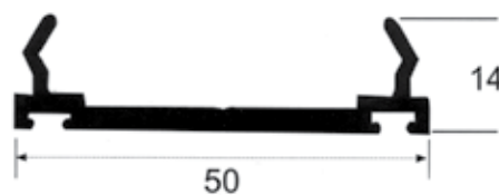
M - 65 0,432 kg/m
