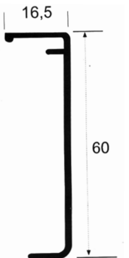
M - 48 0,295 kg/m
